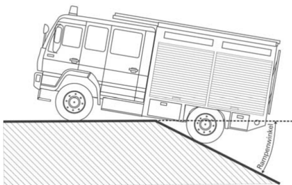
Bild 28: Rampenwinkel
