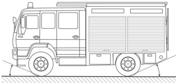
Bild 27: Vorderer und hinterer Überhangwinkel
